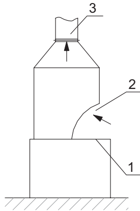
Hình 12.5: Cấu tạo tử hút
