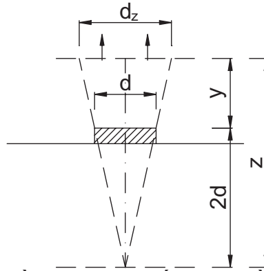
Hình 12.6: Luồng không khí bốc lên từ bề mặt toả nhiệt
