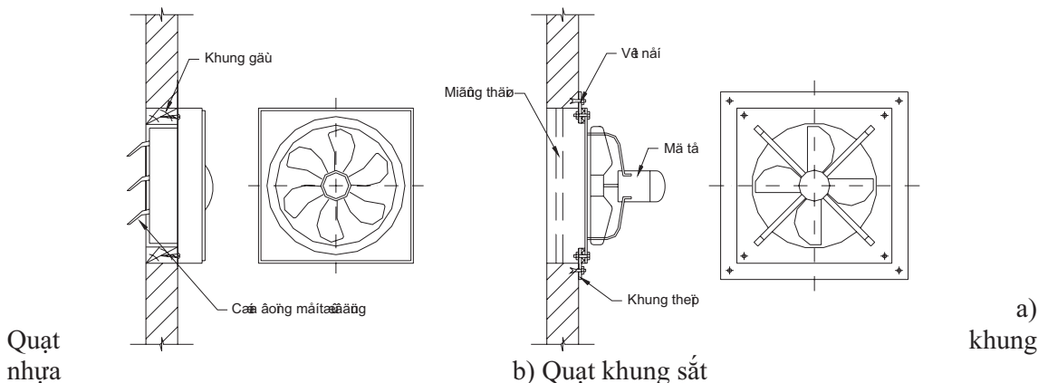
Hình 12.2 : Lắp đặt quạt gắn tường
