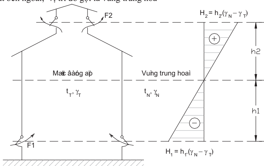
Hình 12.1 : Nguyên lý thông gió do nhiệt áp
